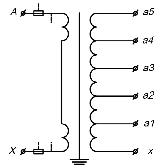
Принципиальная электрическая схема трансформатора ОЛСП-2,5/20
