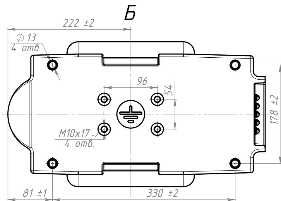
Рис.1 Общий вид трансформатора ОЛС-0,63(1,25)/35
