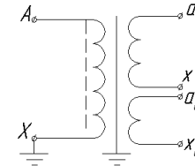
Рисунок А.2 Принципиальная электрическая схема трансформаторов ЗНОЛ
