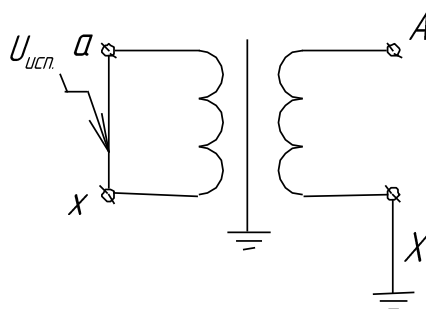
Рисунок Б.3 Схема испытания электрической прочности изоляции вторичной обмотки трансформатора приложенным напряжением 3 кВ промышленной частоты
