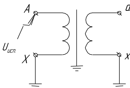
Рисунок Б.2 Схема испытания электрической прочности изоляции первичной обмотки трансформатора приложенным напряжением 1,3 номинального частоты 50 Гц
