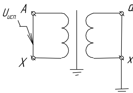
Рисунок Б.4 Схема испытания электрической прочности изоляции первичной обмотки трансформатора приложенным напряжением 85,5 кВ промышленной частоты
