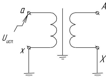
Рисунок Б.1 Схема испытания электрической прочности изоляции первичной обмотки трансформатора индуцированным напряжением частоты 400 Гц
