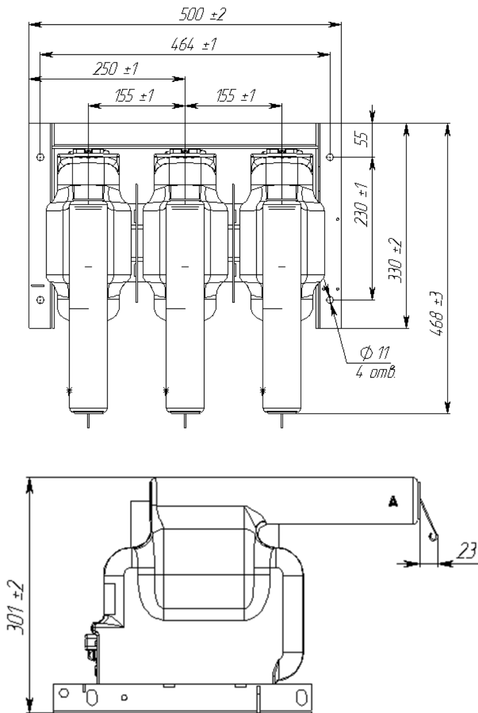
Рисунок А.4 Общий вид трехфазной группы ЗХЗНОЛ.01ПМИ
