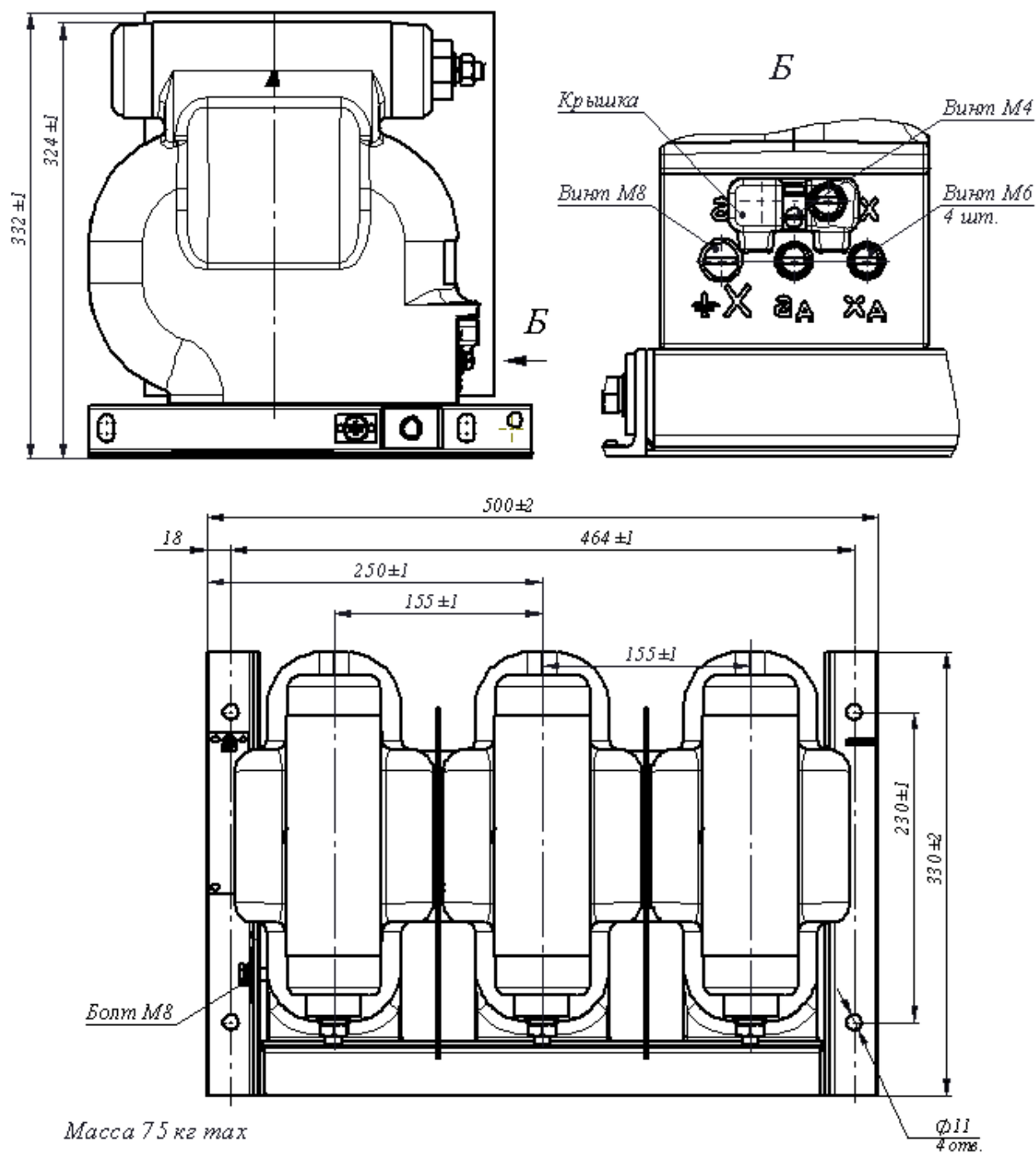
Рисунок А 1 Общий вид трехфазной группы 3x3НОЛПМ
