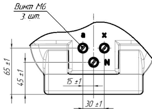
Рисунок А.2 Клеммник трансформатора ТННП
