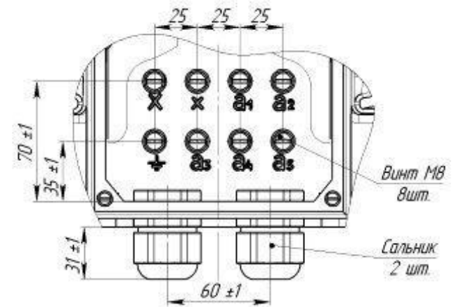
Рисунок А.2 Клемник трансформаторов ОЛЗ-1,25/27,5
