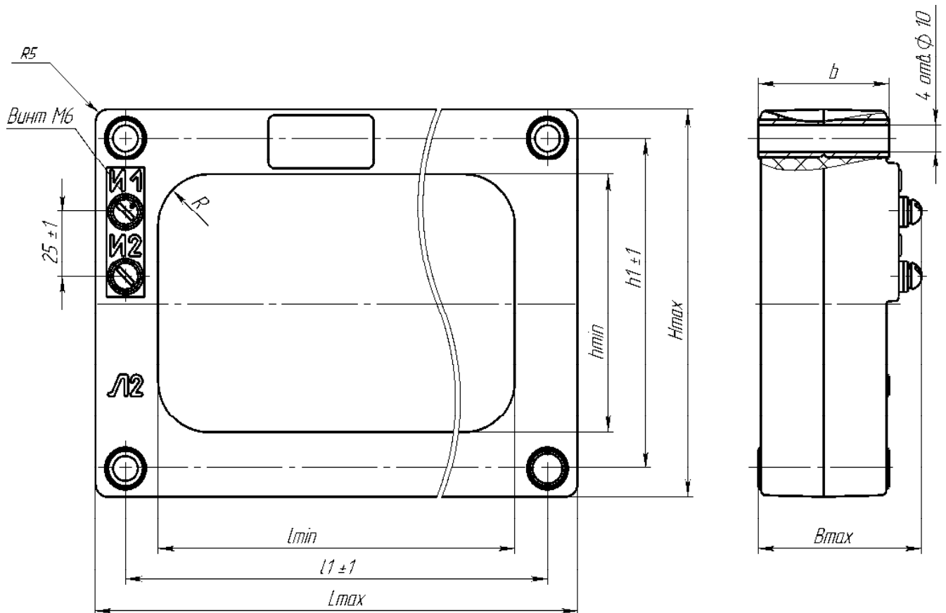
Рисунок А.4 Общий вид трансформаторов ТЗЛМ-100х490, ТЗЛМ-100х590, ТЗЛМ-100х700, ТЗЛМ-250х590, ТЗЛМ-300х590, ТЗЛМ-450х590
