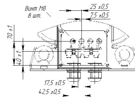
Рисунок А.2 Клемник для трансформаторов ЗНОЛ4-35 III (остальное см. рисунок А.1, крышка условно не показана)
