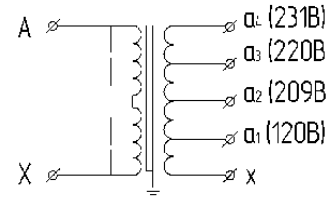
Рисунок А.4 Принципиальная электрическая схема трансформаторов 0/1-0,63/6 (110)/0,12 и 0/1-1,25/6 (110)/0,12
