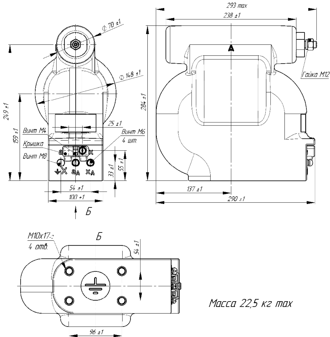
Рисунок Б.1 Внешний вид трансформаторов ЭНОЛПМ
