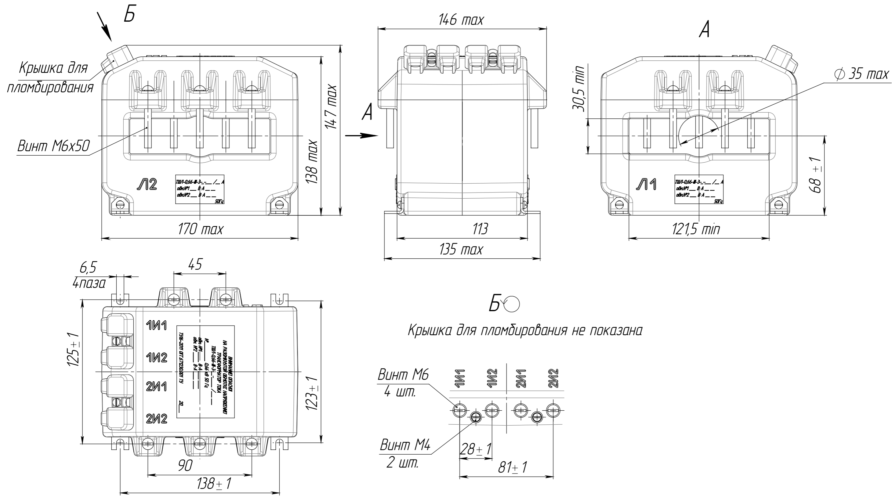
Рис.1. Общий вид трансформатора ТШЛ-0,66-III-3-2
