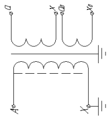
Рисунок А.2 Принципиальная электрическая схема трансформаторов ЗНО/106
