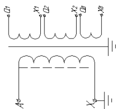
Рисунок А.3 Принципиальная электрическая схема для исполнения ЗНО/106.4
