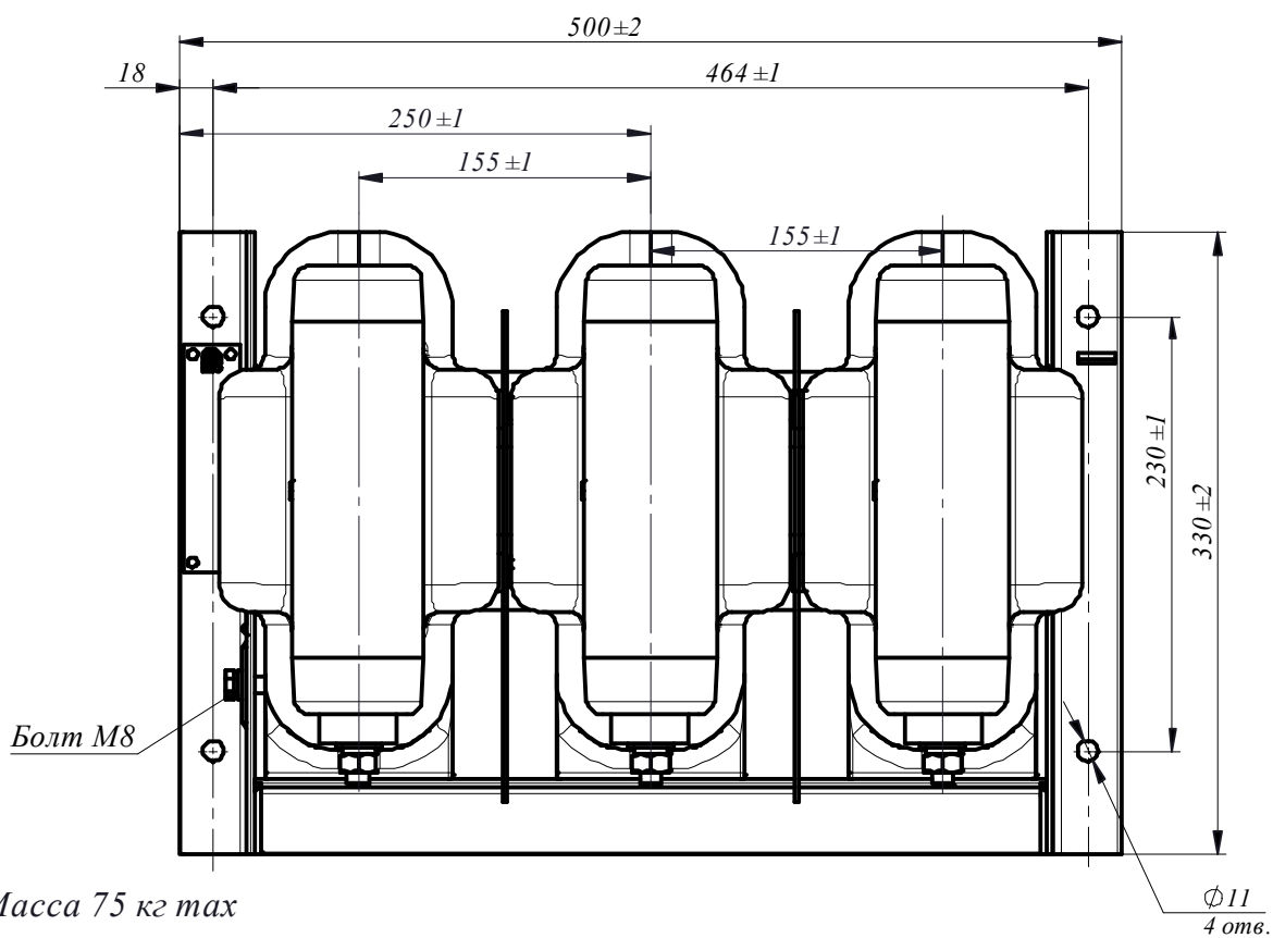
Рисунок А.1 Общий вид трехфазной группы 3хЗНОЛПМ
