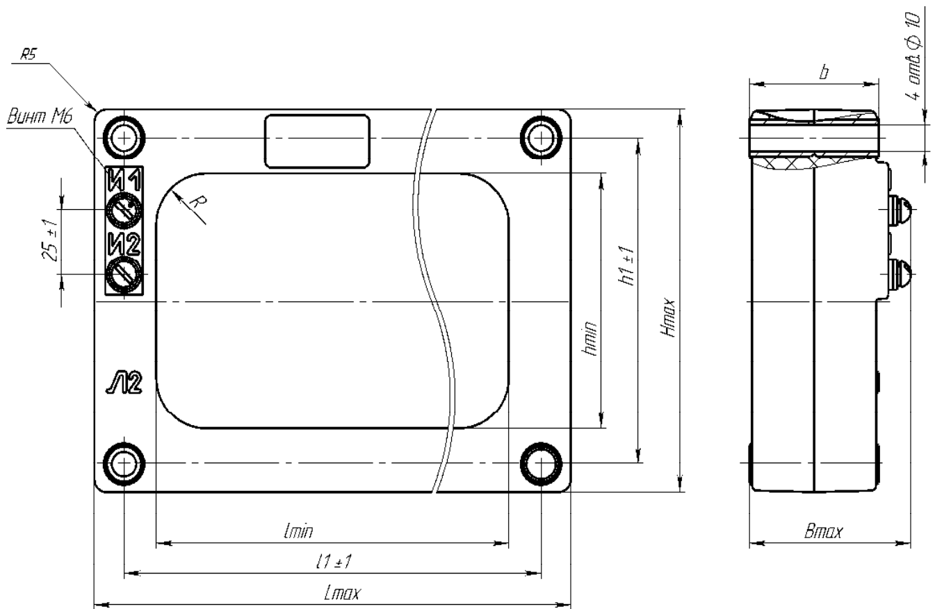
Рисунок А.4 Общий вид трансформаторов ТЗЛМ-100x490, ТЗЛМ-100x590, ТЗЛМ-100x700, ТЗЛМ-250x590, ТЗЛМ-300x590, ТЗЛМ-450x590
