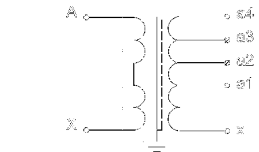
Рисунок Д.2 Принципиальная электрическая схема трансформатора
