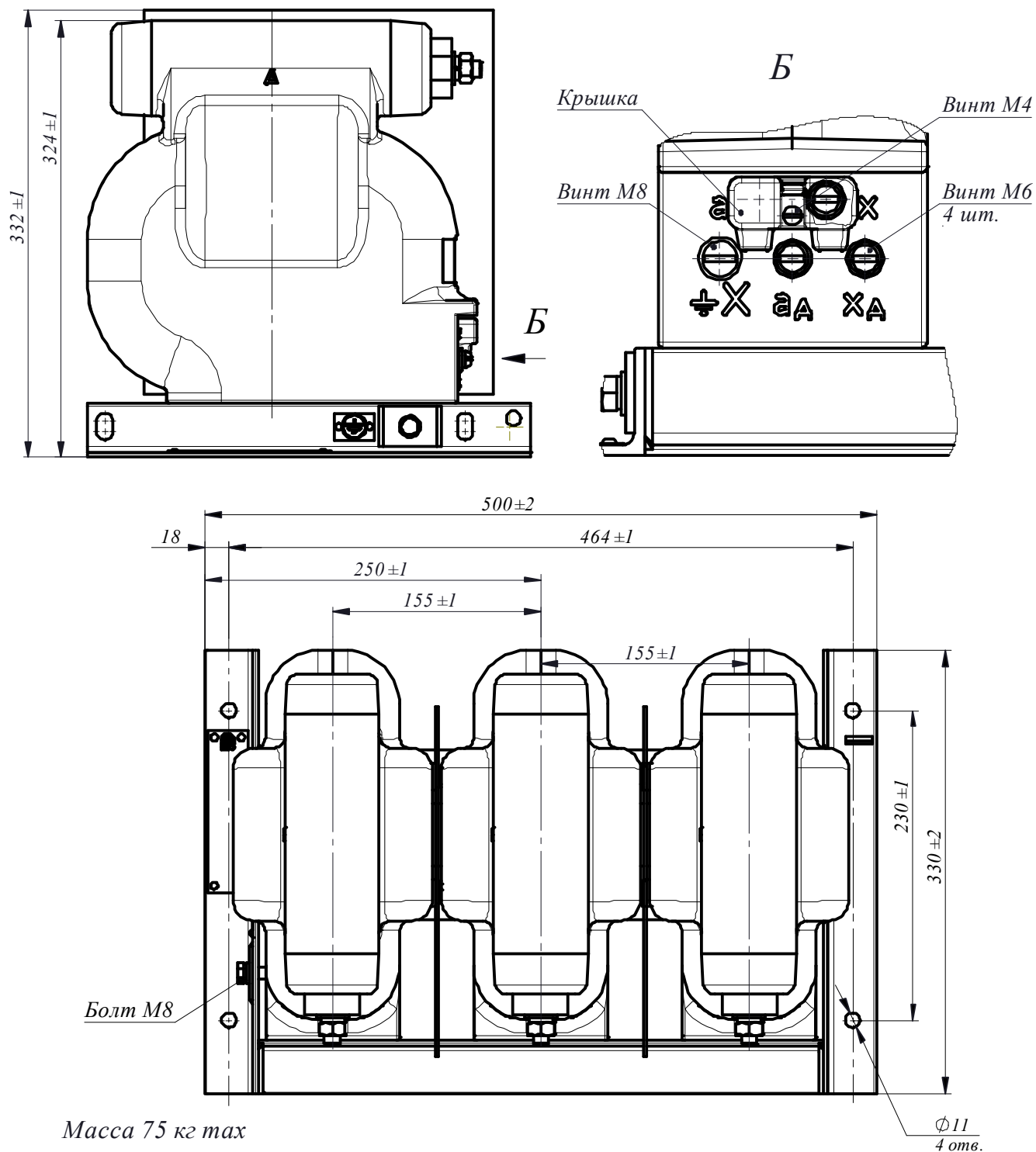
Рисунок А.1 Общий вид трехфазной группы 3хЗНОЛПМ
