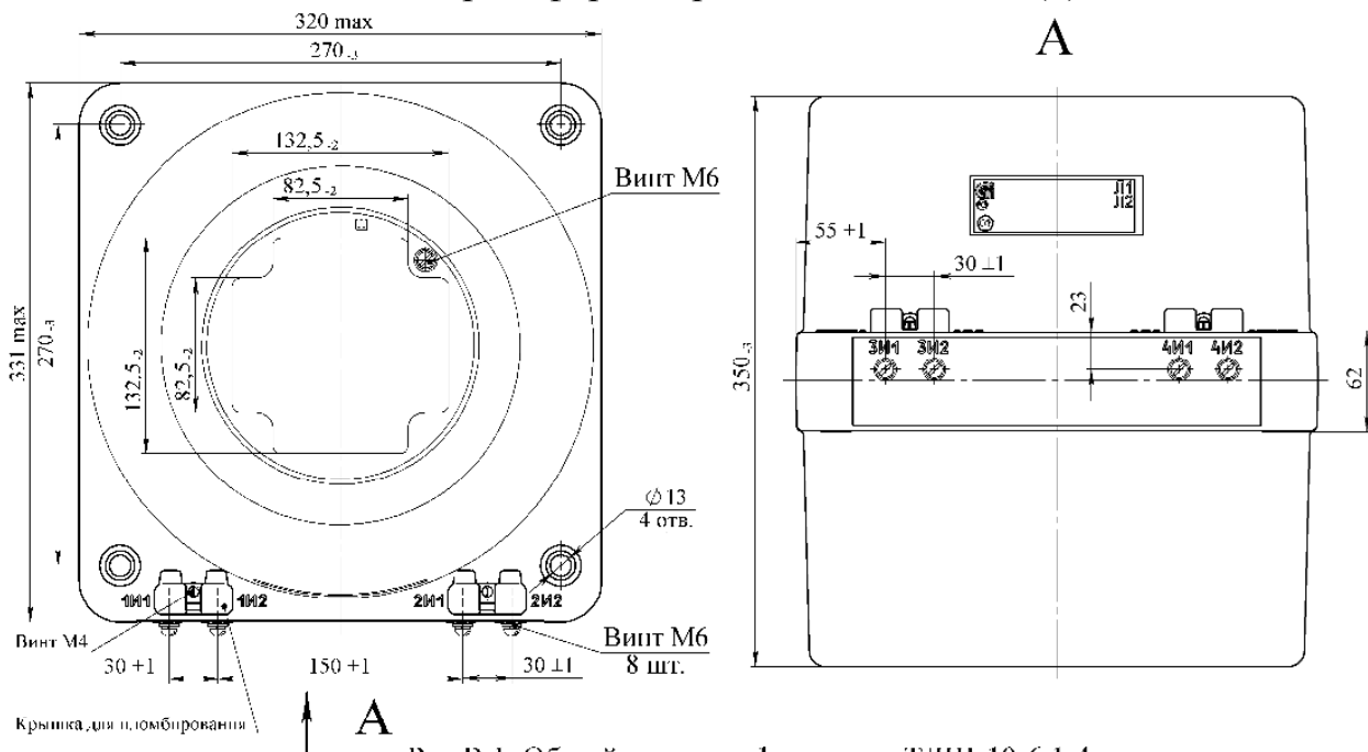
Рис.В.1. Общий вид трансформатора ТЛШ-10-6.1-4
