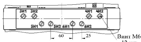
Рис.В.3. Клеммник ТЛШ-10-6.1-6 Остальное см. рис.В.2
