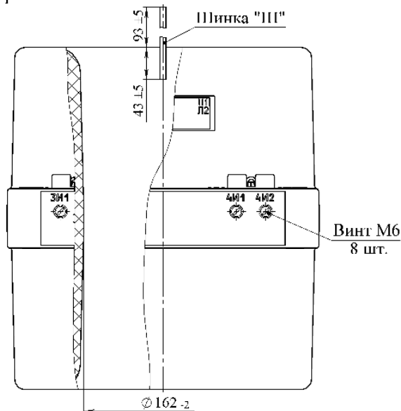
Рис.В.4. Общий вид трансформатора ТЛШ-10-7.1-4 (5,6) Остальное см. рис.В.1,В.2,В.3
