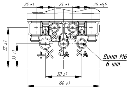
Рисунок А.5 Клемник для исполнения ЗНО/06.4 (остальное см. рисунок А.1)
