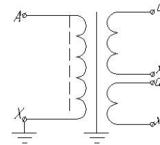
Рисунок А.2 Принципиальная электрическая схема трансформаторов ЗНО/06
