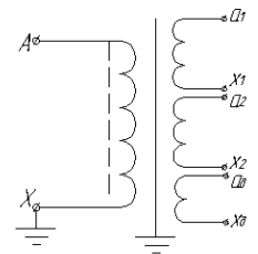
Рисунок А.3 Принципиальная электрическая схема для исполнений ЗНО/06.4
