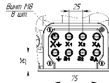
Рисунок А.3 Клемник для трансформаторов ЗНО/ЛО1ПММІ.4-35 (остальное см. рисунок А.1, крышка условно не показана)
