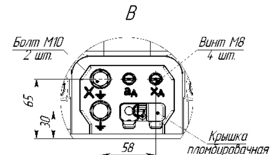
Рисунок А.2 Клемник для трансформатора ЗНО/ЛО1ПММІ-35
