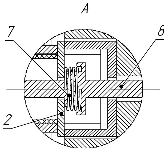
Рисунок В.1 Установка защитного предохранительного устройства в трансформатор ЗНОЛП
