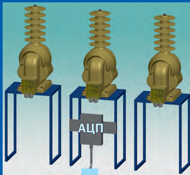
ТРАНСФОРМАТОРЫ НАПРЯЖЕНИЯ
