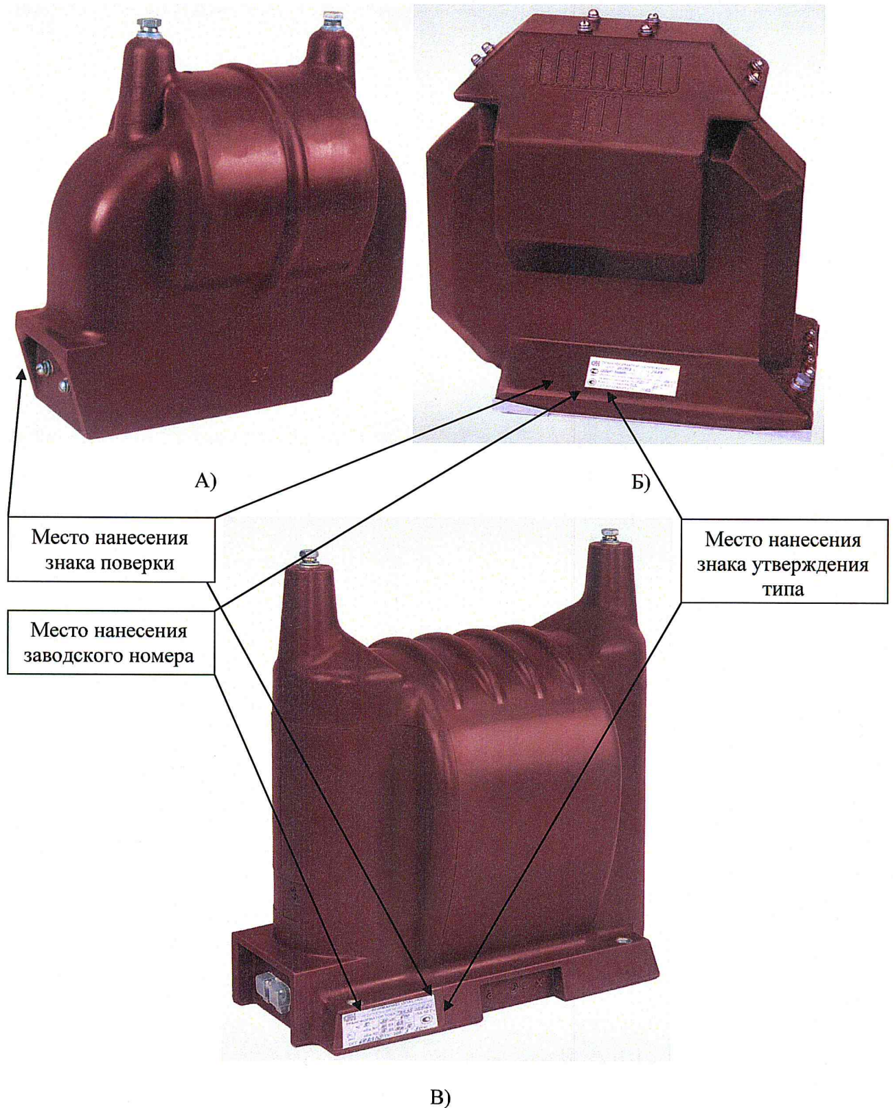
Рисунок 1 - Общий вид трансформаторов напряжения измерительных лабораторных серии НЛЛ: А) НЛЛ-3, НЛЛ-6, НЛЛ-10; Б) НЛЛ-15, НЛЛ-15-1, НЛЛ-15-2, НЛЛ-15-3, НЛЛ-15-4, НЛЛ-35, НЛЛ-35-1, НЛЛ-35-2, НЛЛ-35-3, НЛЛ-35-4, НЛЛ-35-5; В) НЛЛ-35-6. Общий вид таблички, места нанесения заводского номера, места нанесения знака утверждения типа и знака поверки
